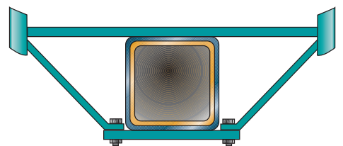
Der doppelwandige Zentralholm ist für höchste Belastungen ausgelegt
